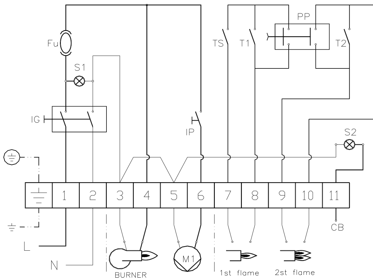
Рис. 4 – Схема подсоединения 2-ступенчатой горелки
