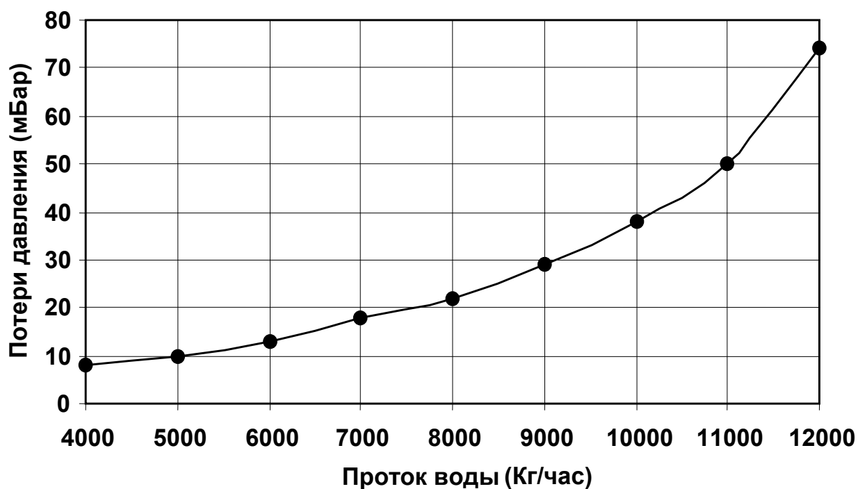
ПОТЕРИ ДАВЛЕНИЯ КОТЛА 110 (150, 195, 220) NL
